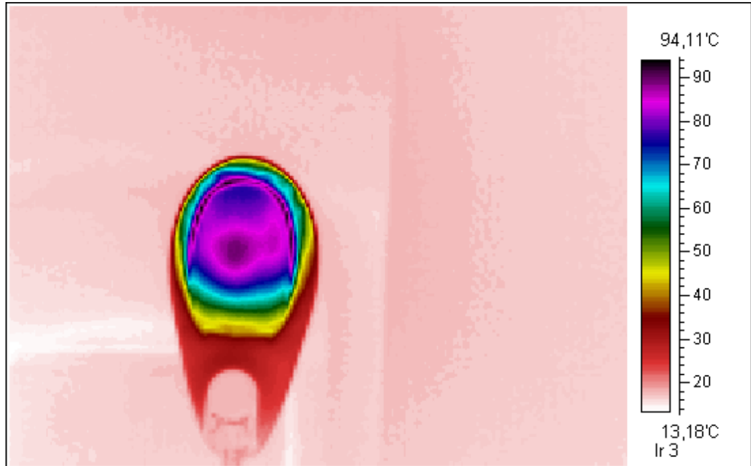
Analiza termografica dupa 3:00h de fct. - CITADIN + Philips SON-T 250W
