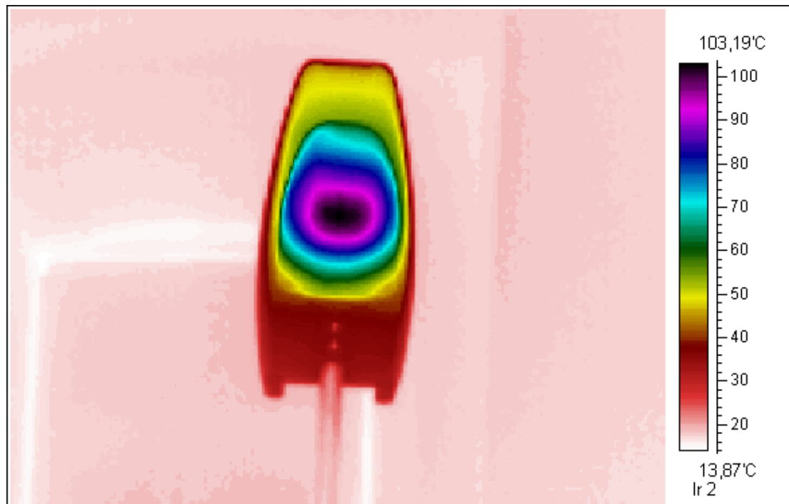
Analiza termografica dupa 3 h AMBAR3 + OSRAM NAV-T 250W Tmax=103,33 Grd.; Tamb=19,2 Grd.; Umid=56,2%
